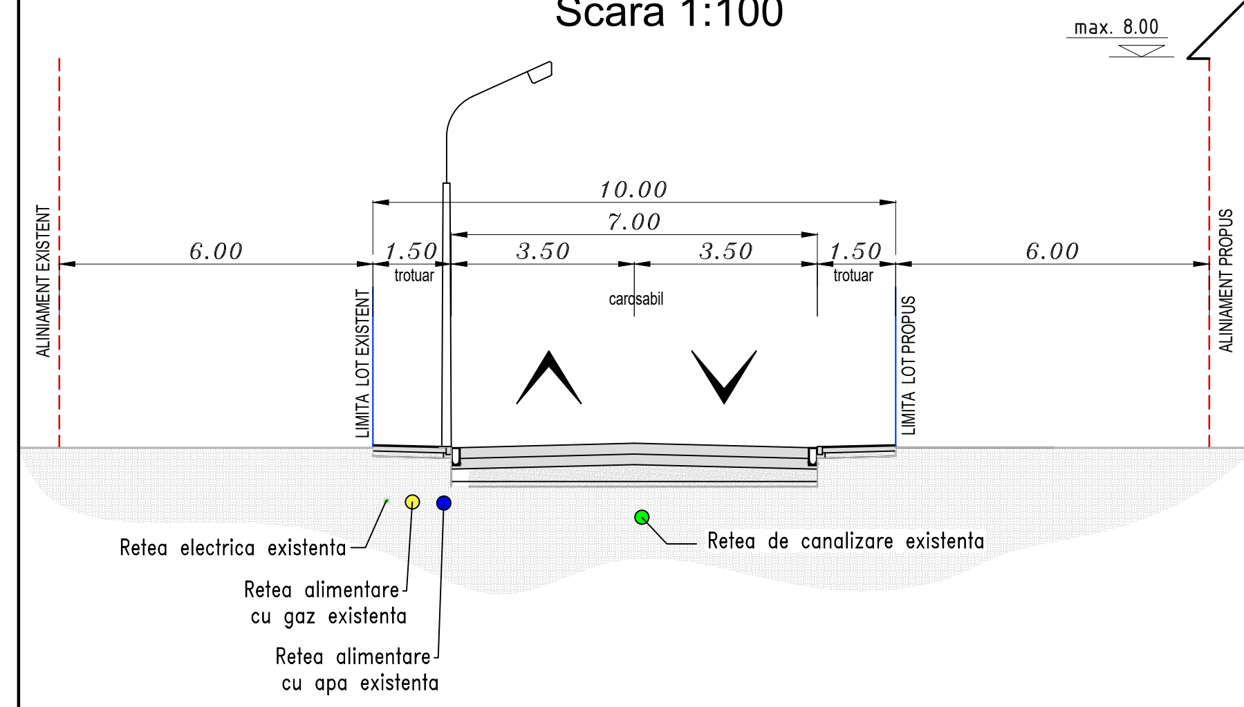
B PROFIL STRADAL PROPUZ Scara 1:100
