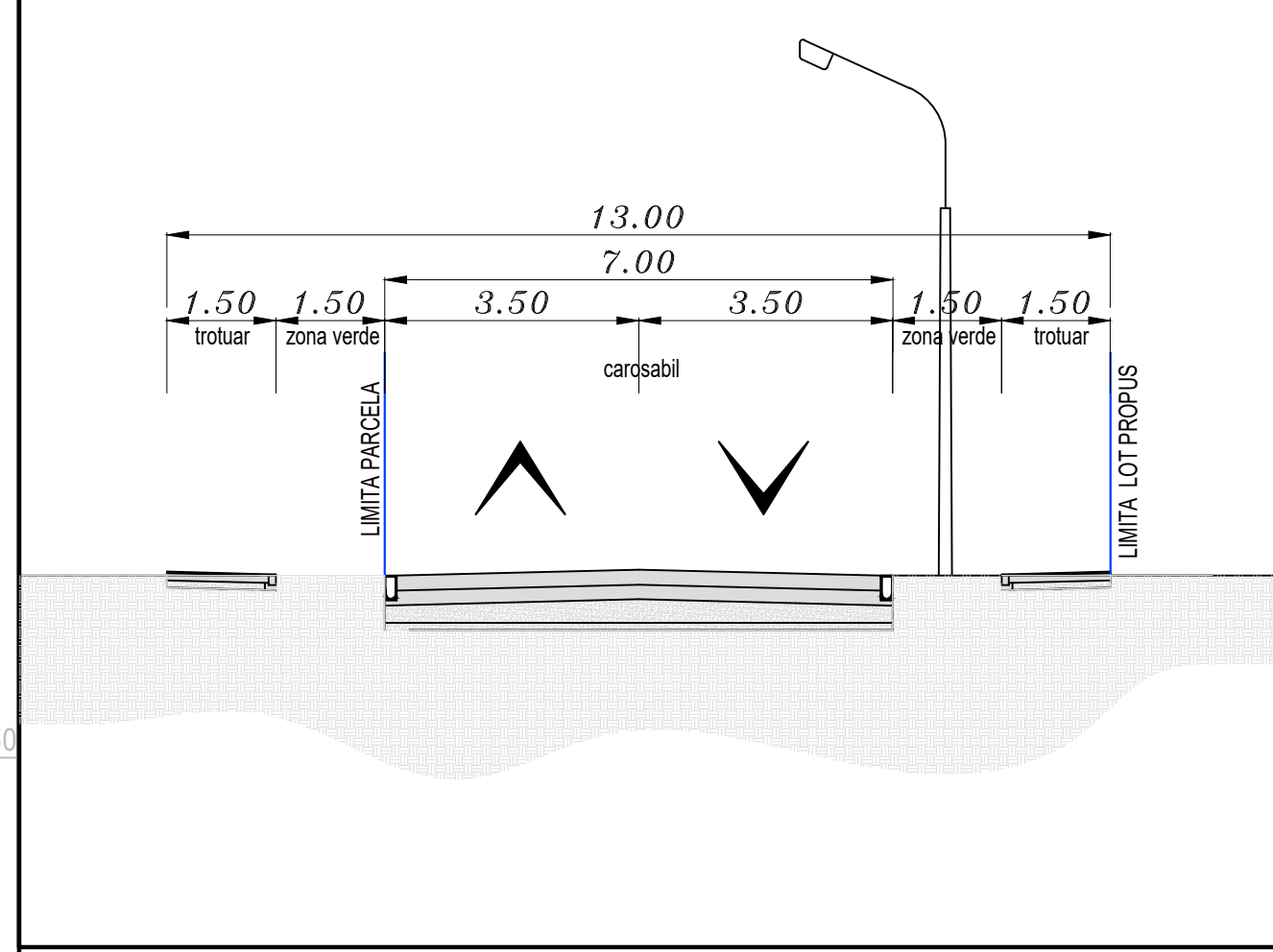
B PROFIL STRADAL PROPUZ Scara 1:100
