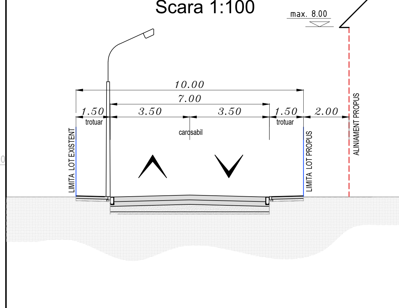
B PROFIL STRADAL PROPUZ Scara 1:100
