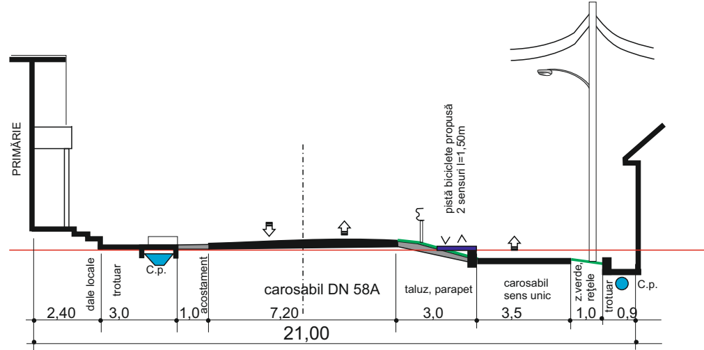
EZERIȘ zona centrală DN 58A sc. 1:250
