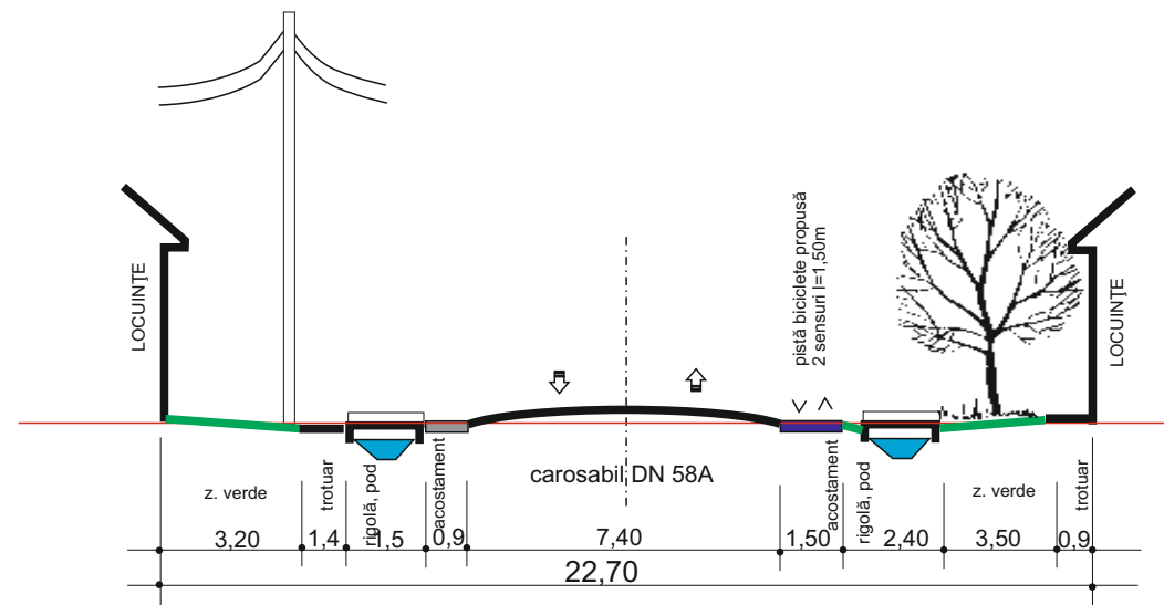
SOCENI zona centrală DN 58 sc. 1:250
