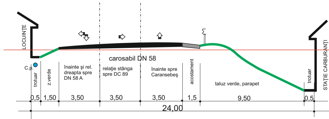
SOCENI zona centrală DN 58 sc. 1:250
