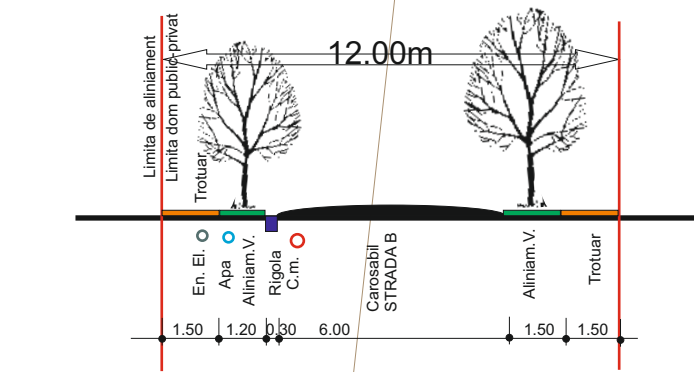
PROFIL STR. B
