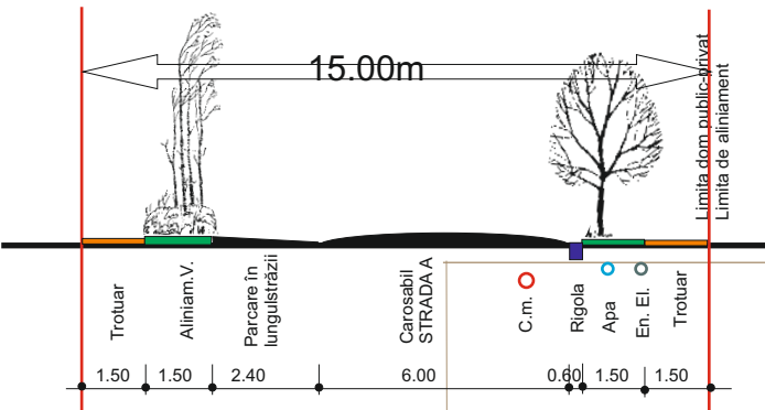
PROFIL STR. A
