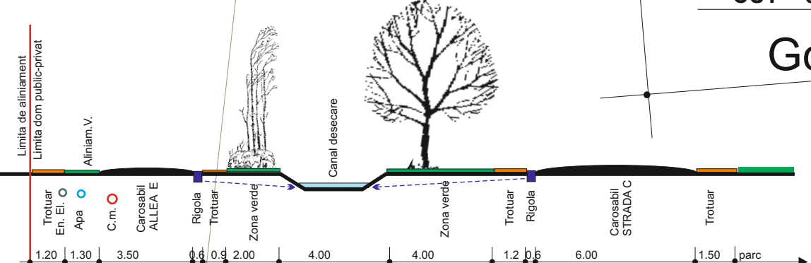
PROFIL AL. E și STR. C
